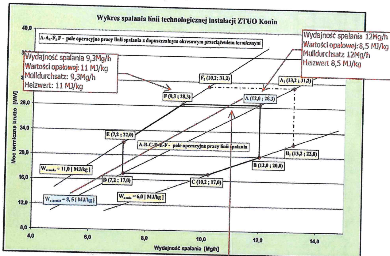
Rysunek 2. Wykres spalania dla linii technologicznej ZTUO.
